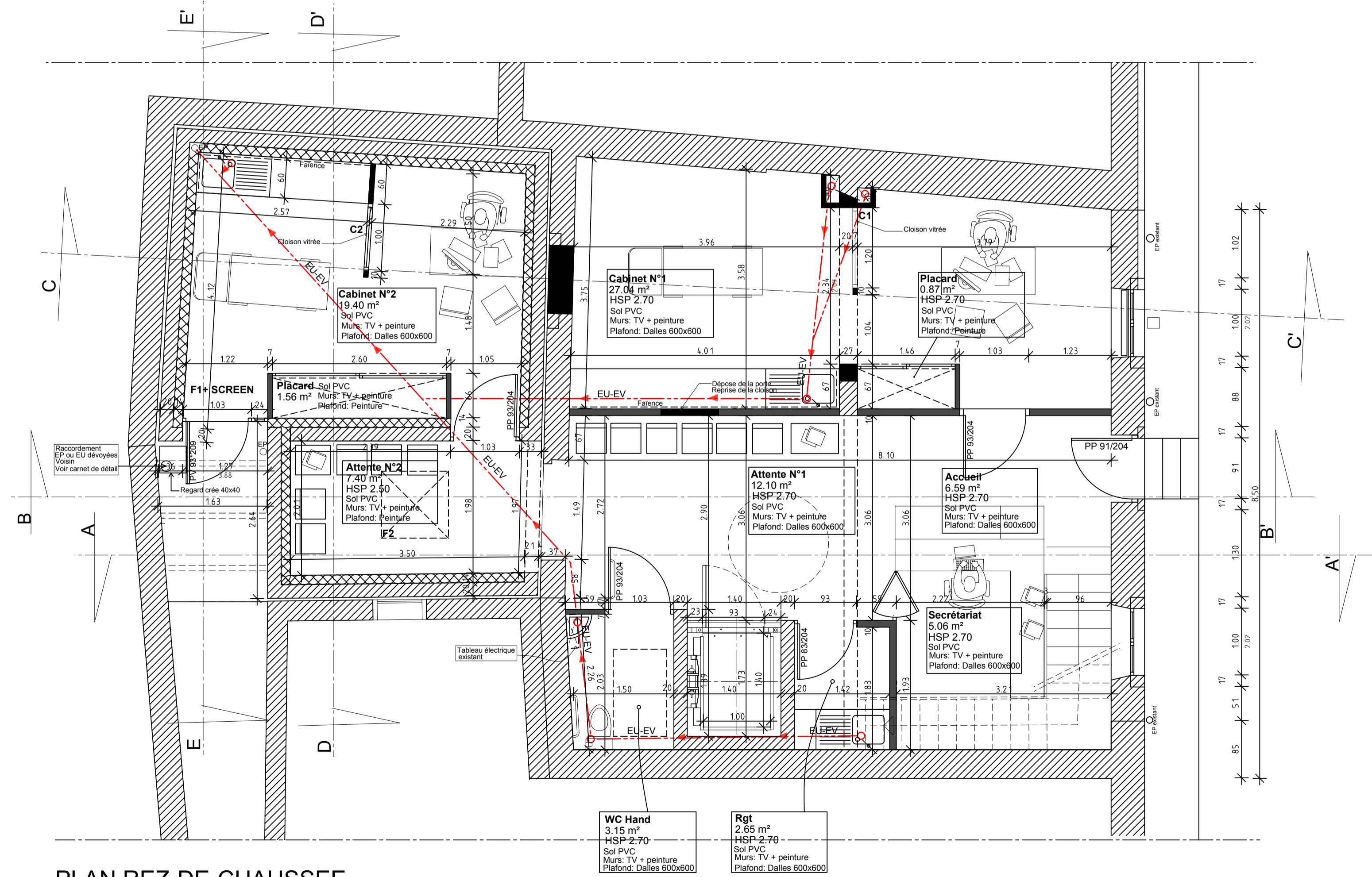
PLAN REZ-DE-CHAUSSEE
