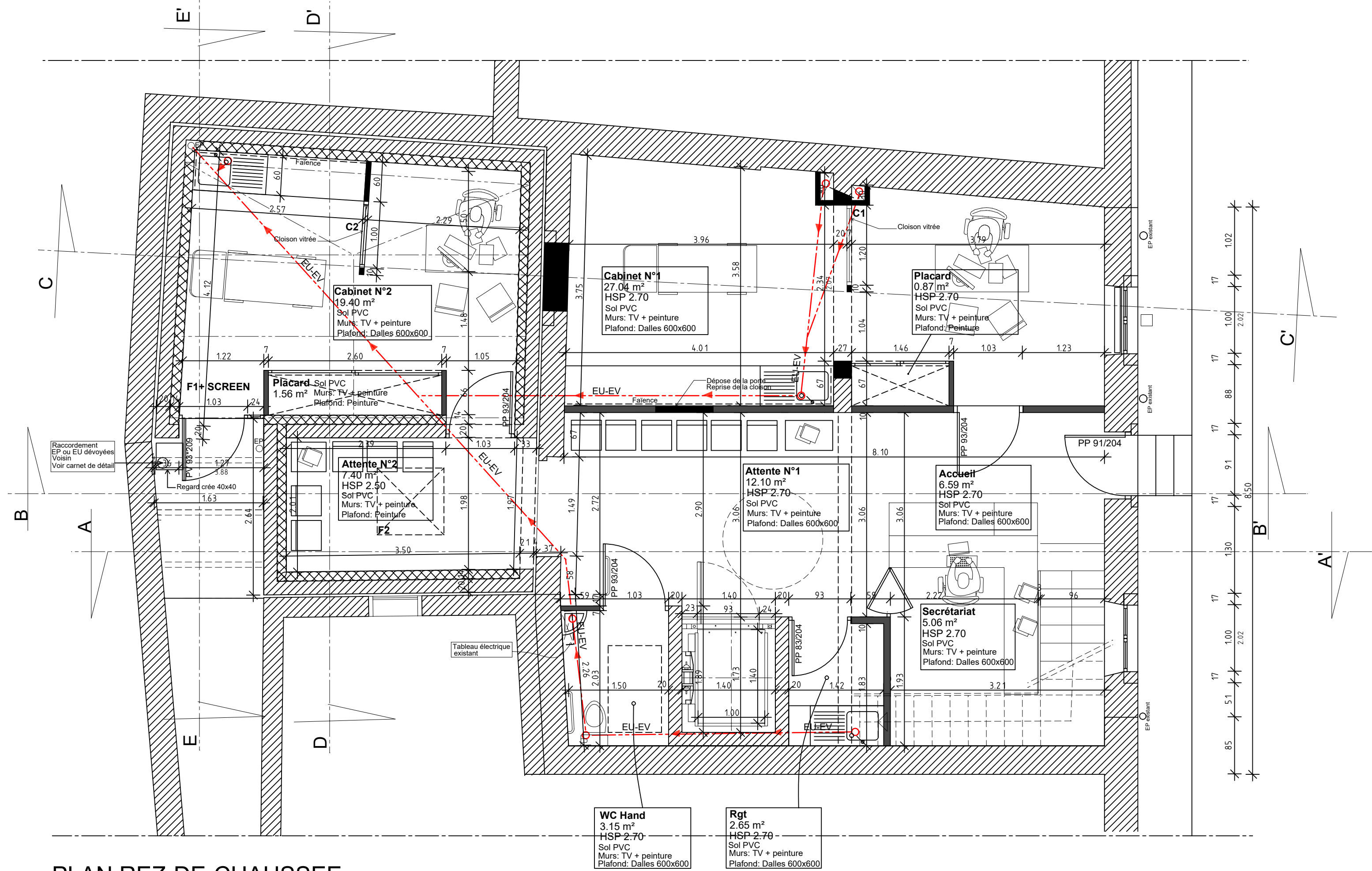
PLAN REZ-DE-CHAUSSEE
